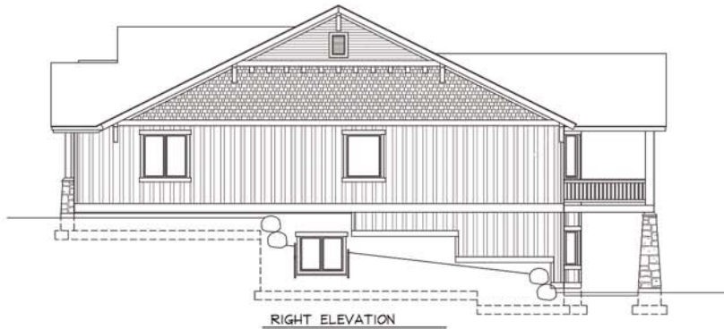
RIGHT ELEVATION
